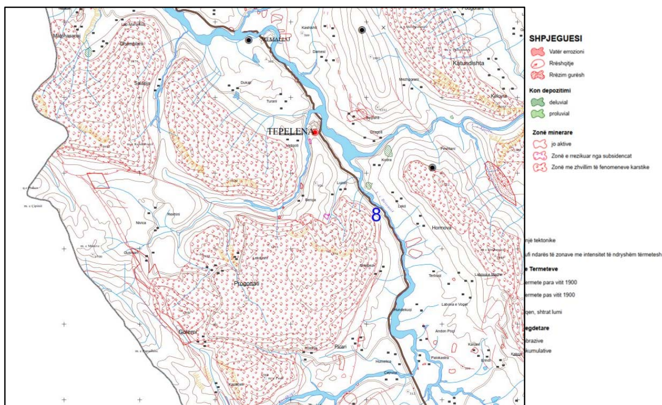
Fig.- Harta e Rrezikut Gjeologjik, Tepelenë
