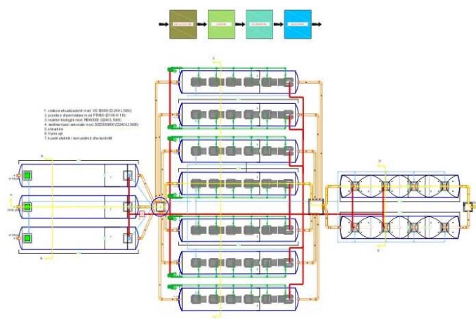
Fig. – Skemë e impiantit të trajtimit të ujrave të zeza
