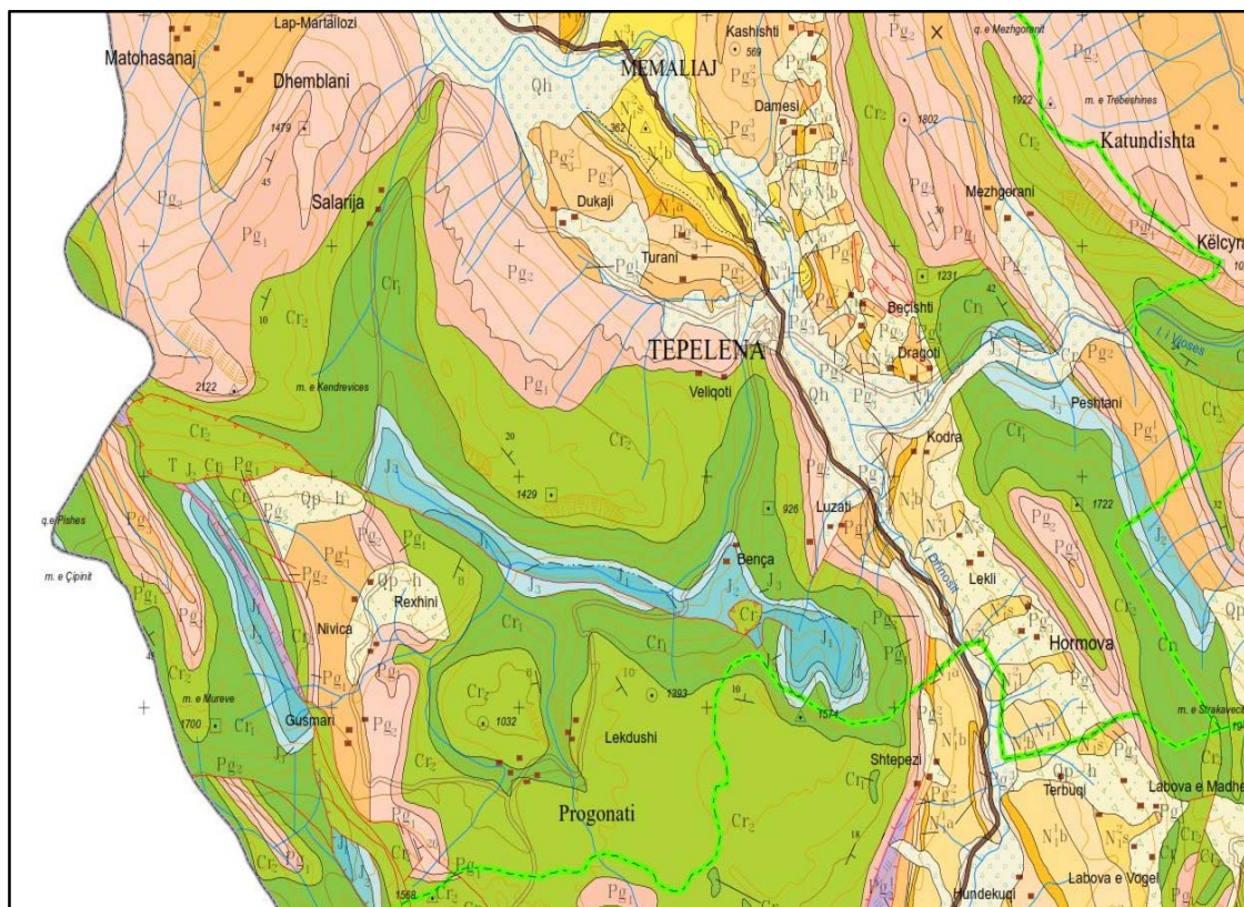
Fig. – Harta Gjeologjike e Bashkisë Tepelenë, shk. 1:100,000 (Burimi: Shërbimi Gjeologjik Shqiptar)
